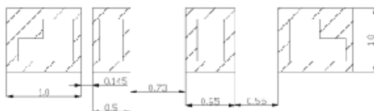
建议焊盘尺寸图:
